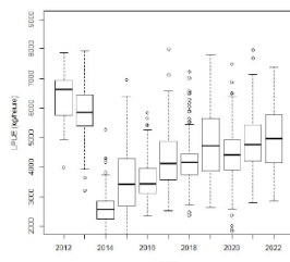
Evolution des rendements horaires du mois de juin entre 2012 & 2022 (zone 5)
