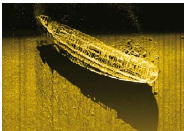
Image sonar du Saint-Dominique (1897).
