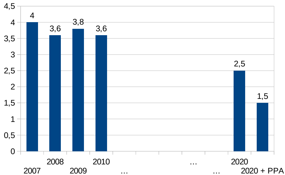
Nombre d'habitants concernés par un dépassement de la valeur limite annuelle du NO2
