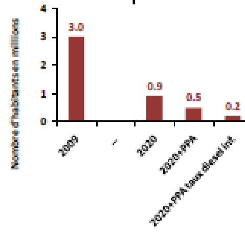
Nombre d'habitants concernés par un dépassement de la valeur limite journalière des PM 2.5
