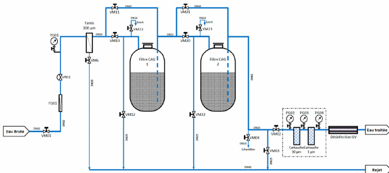
PID DE L'INSTALLATION DE TRAITEMENT
