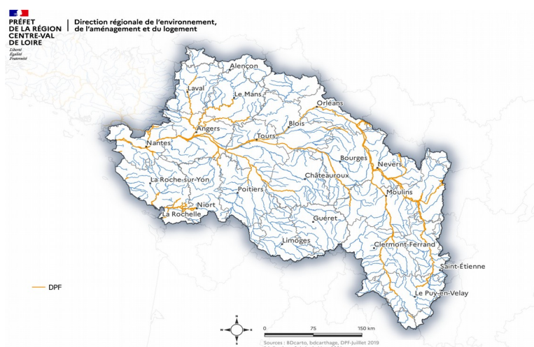
Figure 17 : Domaine public fluvial sur le territoire du PLAGEPOMI et zoom sur le secteur de la Sèvre niortaise
