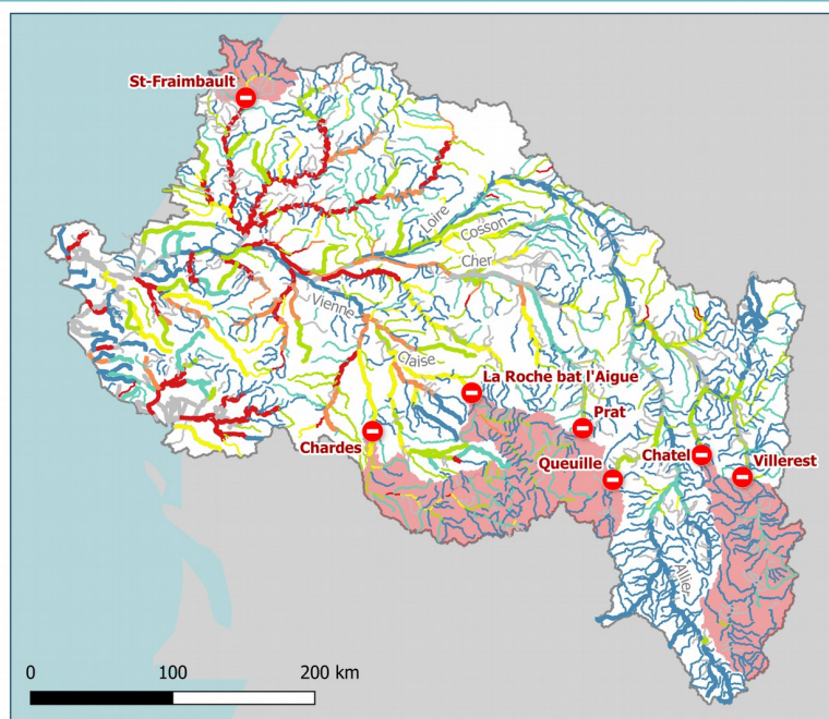
Figure 6 : Taux d'étagement (effet retenue) des masses d'eau correspondant aux axes « Migrateurs » du SDAGE Loire-Bretagne (source : Données OFB 2019, Réalisation : LOGRAMI, 2020)
