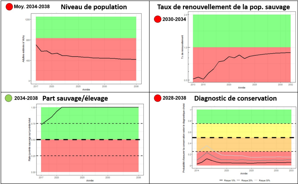
Simulation à 20 ans des 4 indicateurs du PLAGEPOMI pour le saumon atlantique en amont de Vichy sous l'hypothèse d'un arrêt des déversements, d'une suppression des effets négatifs liés aux ouvrages à l'écoulement à la montaison et à la suppression des mortalités dans les ouvrages hydroélectriques lors de la dévalaison (source : Legrand et Prévost, 2020).
