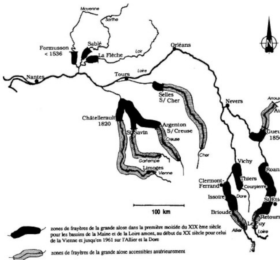
Figure 43 : Répartition ancienne des zones de frayères de la grande alose sur le bassin de la Loire d'après Duhamel du Monceau (1772), Ivolas (1893), Ivoy de la Poype (1901), Benardeau (1905), Angot (1906), Roule (1923), Le Clerc (1941), Salvert (1984), et Poitrineau (1985).
