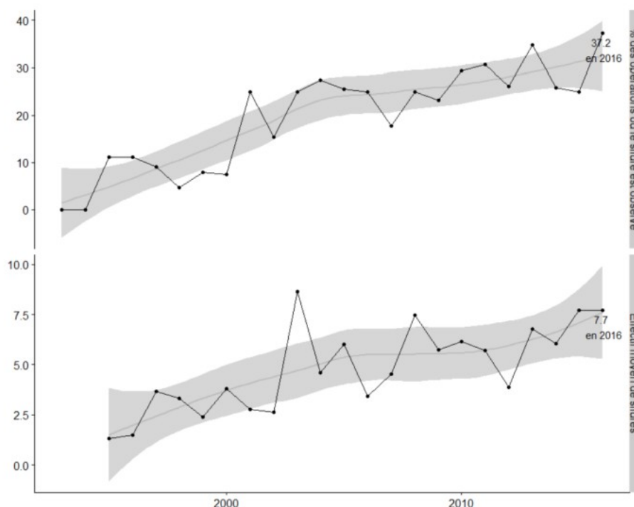
Figure 14 : Évolution interannuelle du % des opérations où le silure a été observé, et de l'effectif moyen de silures par opération de pêche de la BD MAP pour le bassin Loire-Bretagne (protocoles « Grands milieux » et « stratifiés par ambiance ») (source : Données BD MAP/AFB 2018 – Réalisation : Tableaux de Bord Migrateurs, 2019).
